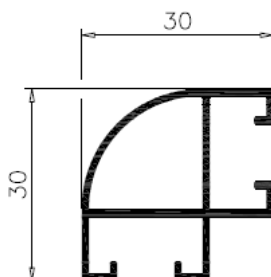
REF. 0166 PESO: 0.394 PERIM.: 264 ESP.: 1.1
