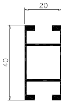
REF. 0165 PESO: 0.486 PERIM.: 266 ESP.: 1.1
