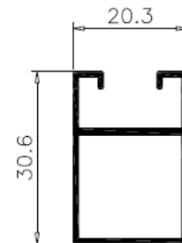
REF. 0164 PESO: 0.327 PERIM.: 219 ESP.: 1.1
