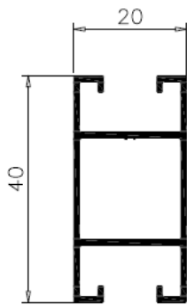
REF. 1.198 PESO: 0.416 PERIM.: 277 ESP.: 1.1
