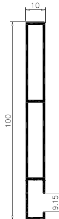
REF. 1.285 PESO: 0.805 PERIM.: 437 ESP.: 1.35
