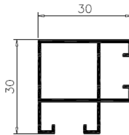
REF. 0163 PESO: 0.418 PERIM.: 280 ESP.: 1.1
