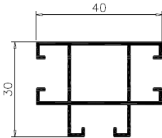
REF. 0162 PESO: 0.513 PERIM.: 344 ESP.: 1.1
