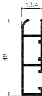
REF. 1.110 PESO: 0.478 PERIM.: 252 ESP.: 1.4
